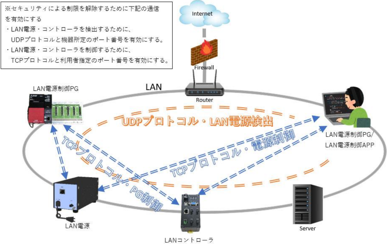
Ethernetで利用するLAN電源・コントローラのネットワーク図
